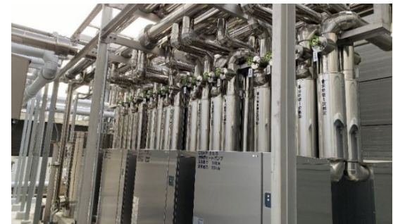
導入したヒートポンプ
