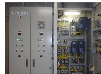
給排気ファンのインバータ制御
