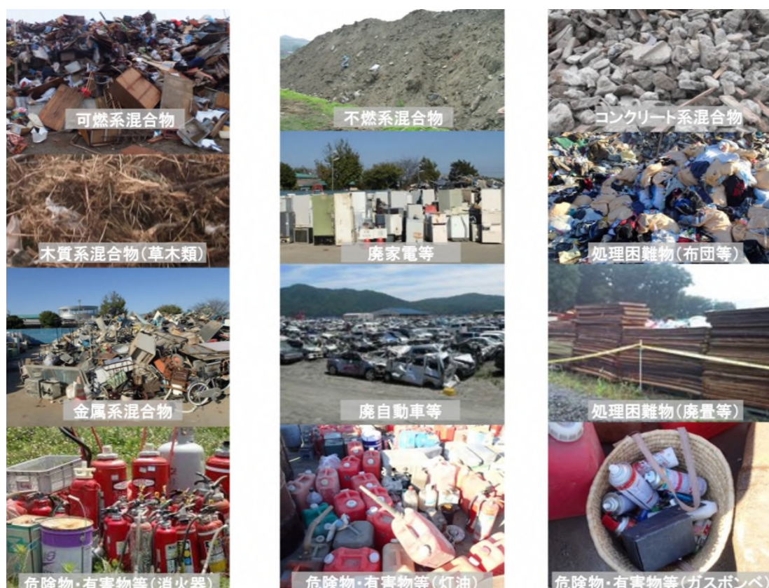
図 1-4-11 一次仮置場の分別例
