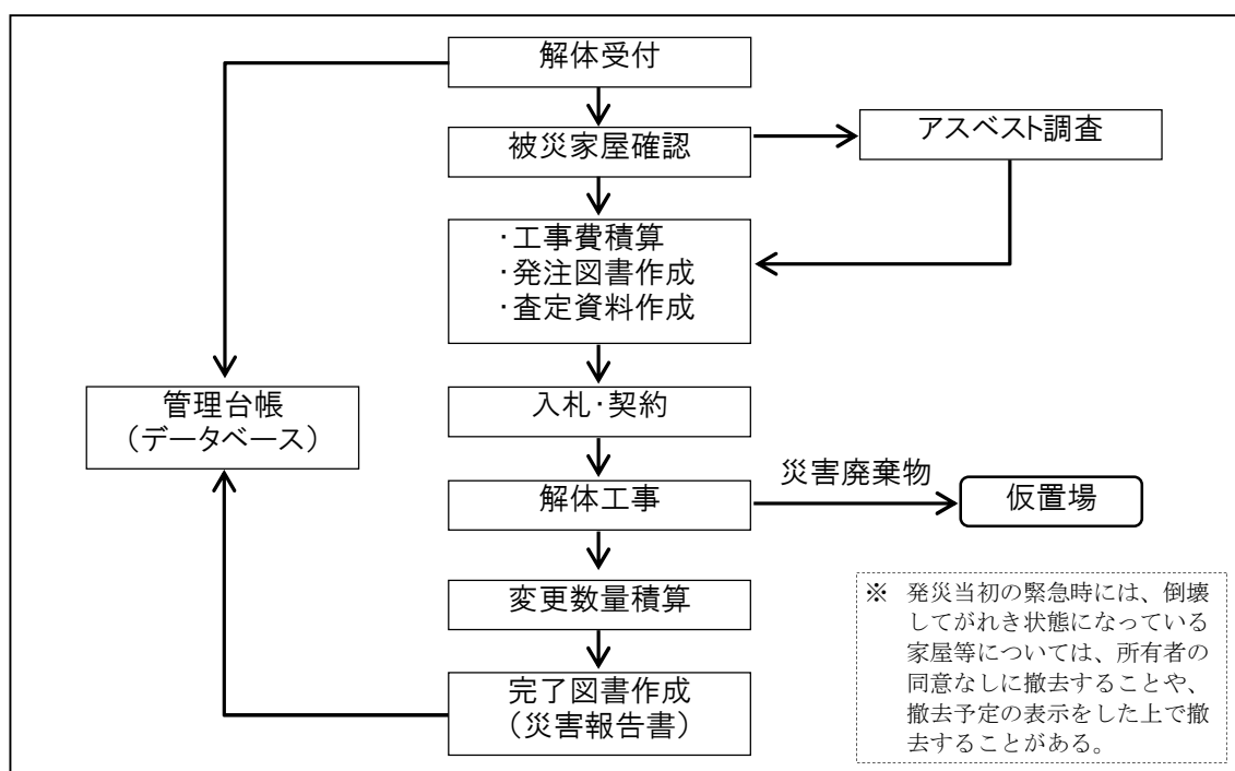
図 1-4-8 損壊家屋等の解体撤去の流れ
