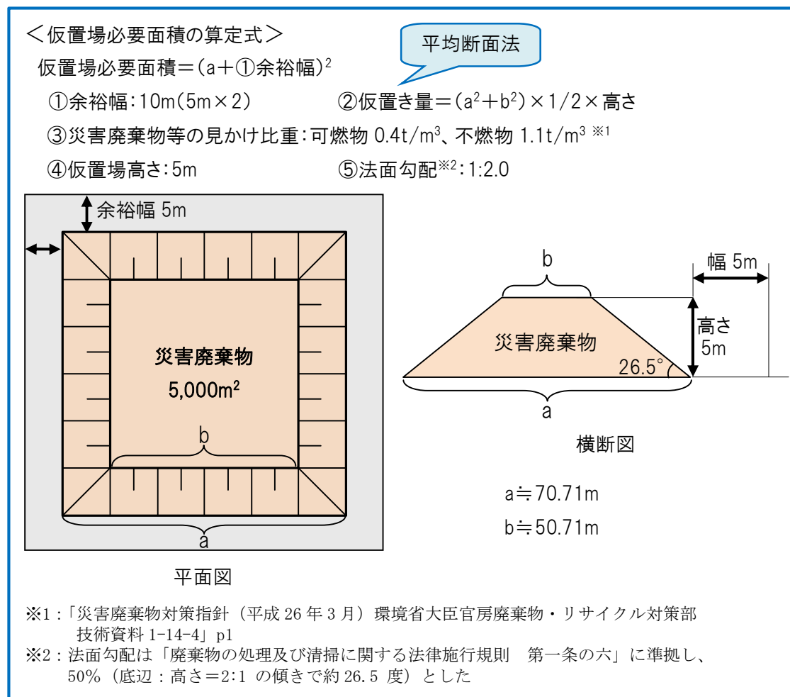
図 5-2-1 一次仮置場面積算定式と模式図
