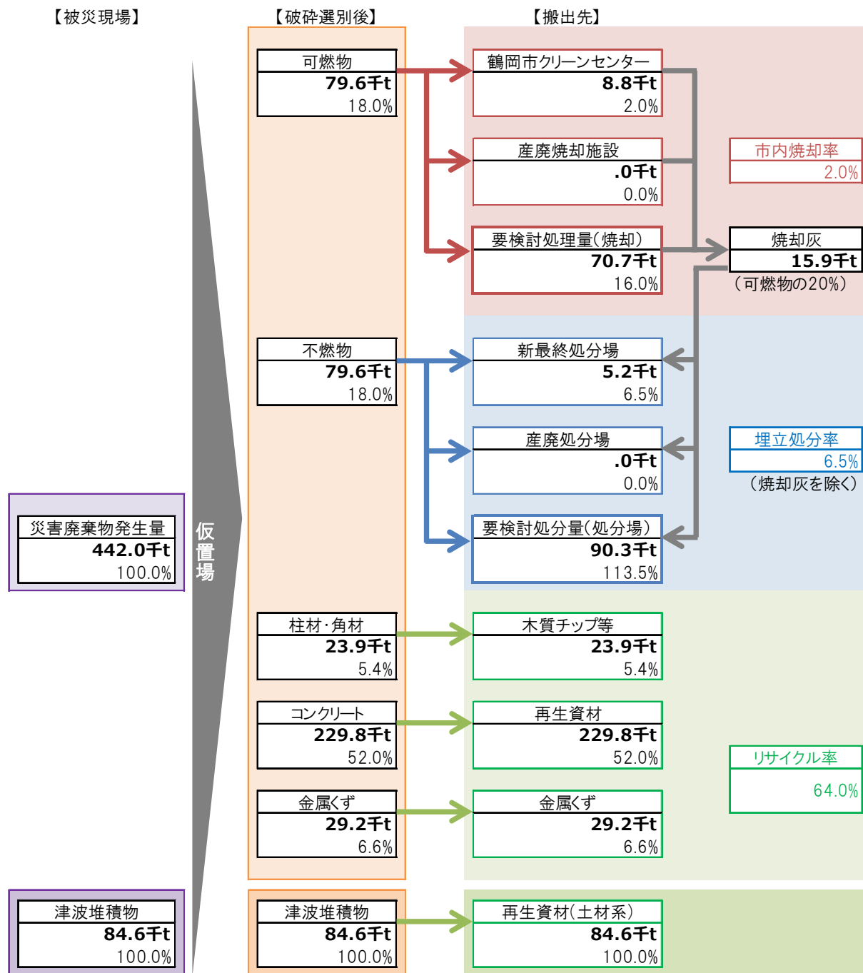
図 4-4-2 主に庄内地域に被害が集中し、三川町、鶴岡市とも被災する場合の処理フロー
