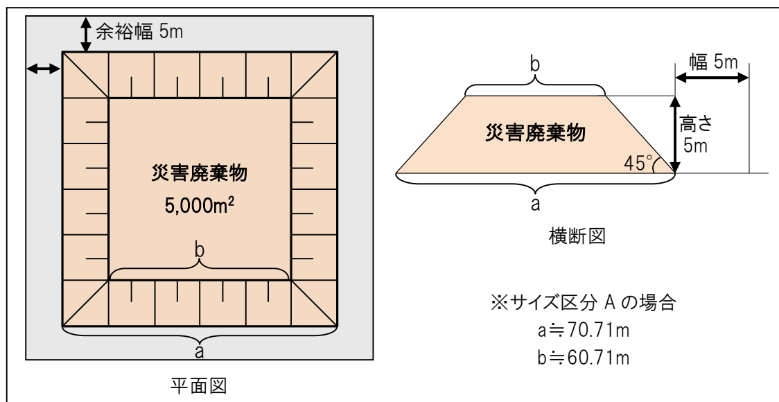
図 1-4-10 仮置きの模式図
